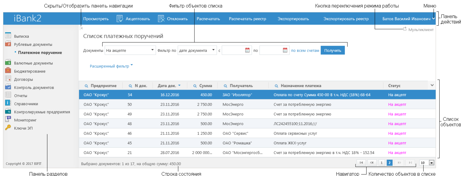
Рис. 1. АРМ "ЦФК". Подраздел "Платежное поручение"
